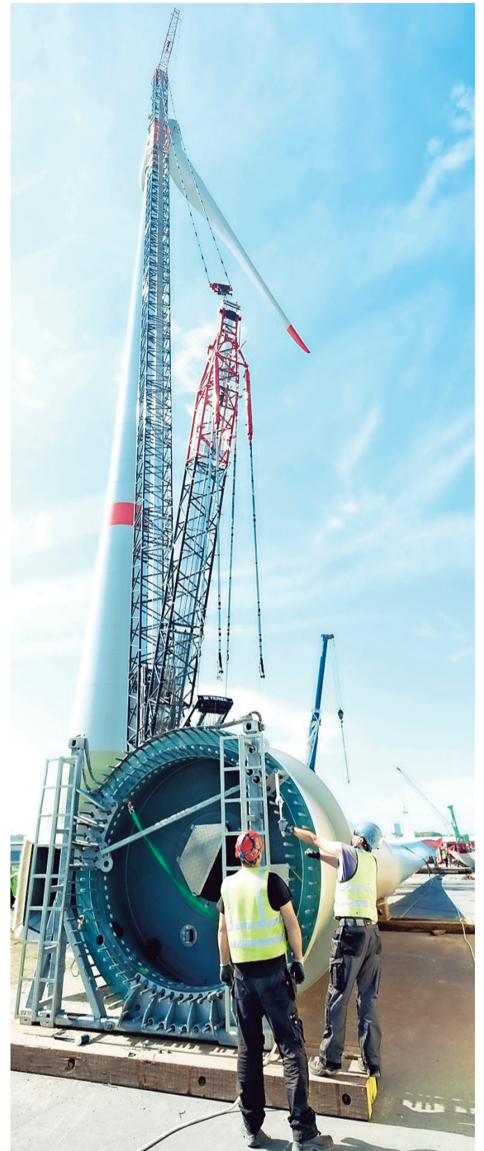
Een wijk, 25 ton zwaar, ligt aan de voet van een toren, klaar om opgehesen te worden. Foto Dirk Laenen
